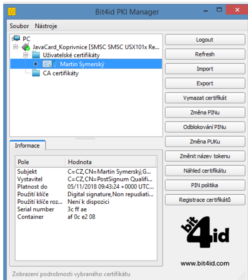
Obrázek 145 - Token - Detail
