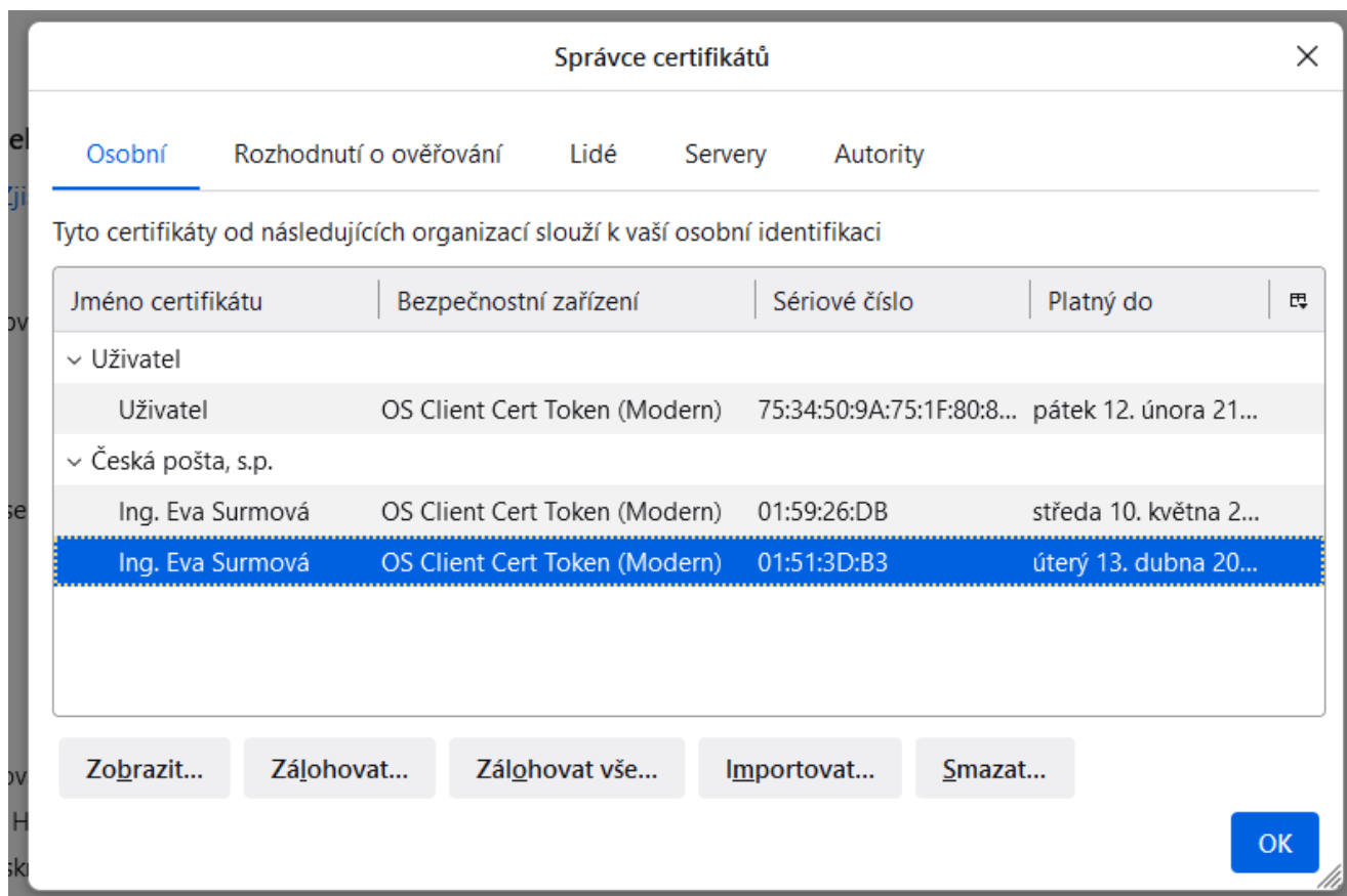
Obrázek 120: Správce certifikátů
