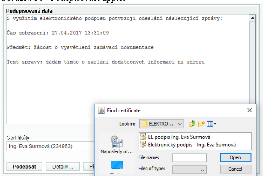
Obrázek 16 - Podepisovací applet
