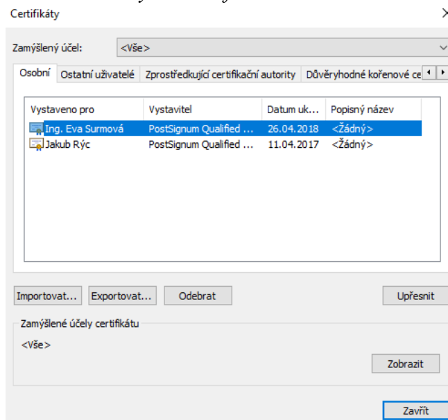
Obrázek 18 - Výběr certifikátu
