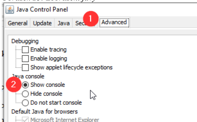
Obrázek 23: Zobrazení javy
