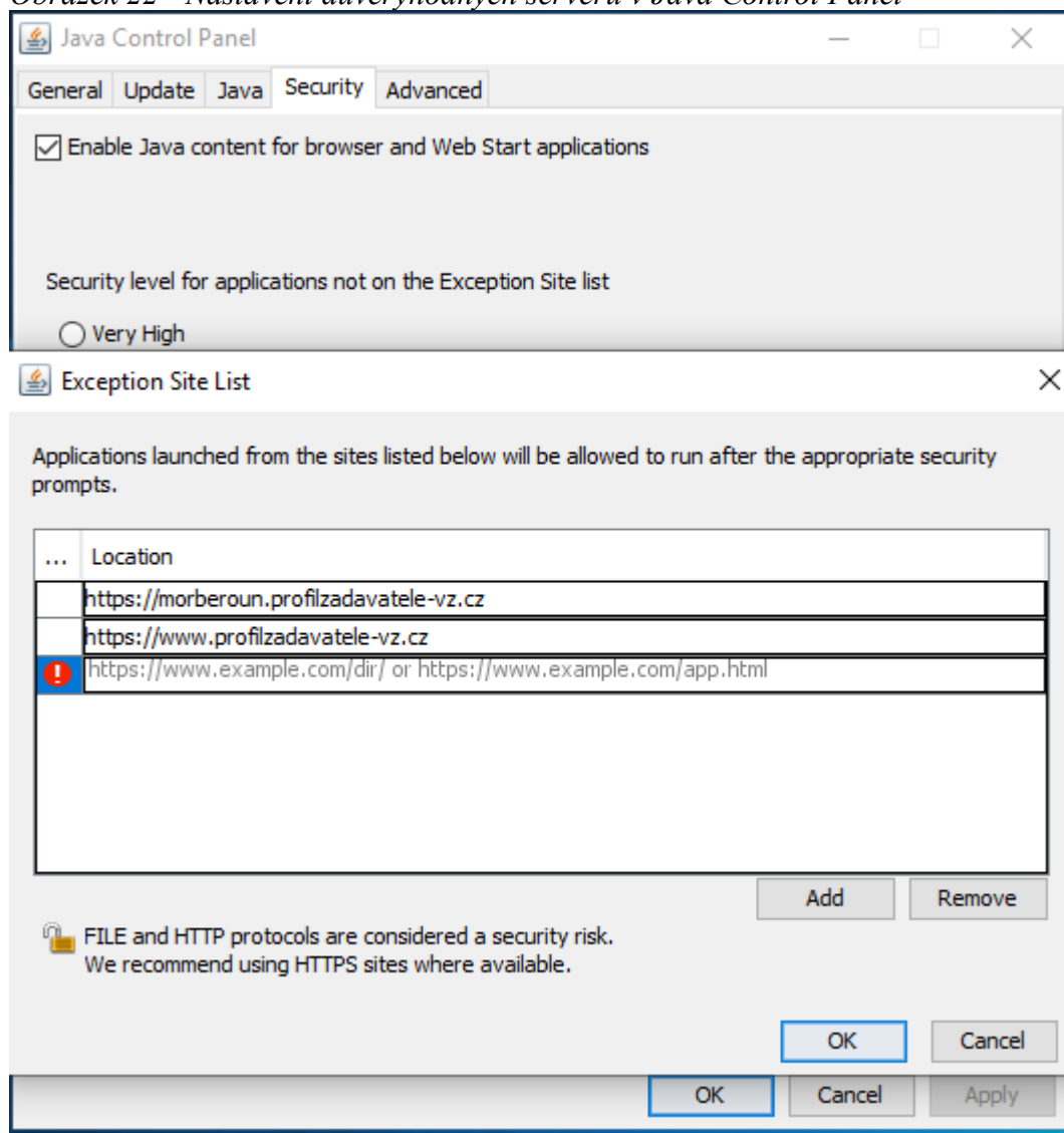
Obrázek 22 - Nastavení důvěryhodných serverů v Java Control Panel
